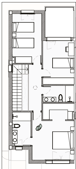
PLANTA PRIMERA
