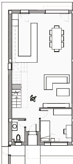
PLANTA BAJA
