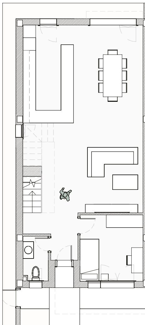
PLANTA BAJA
