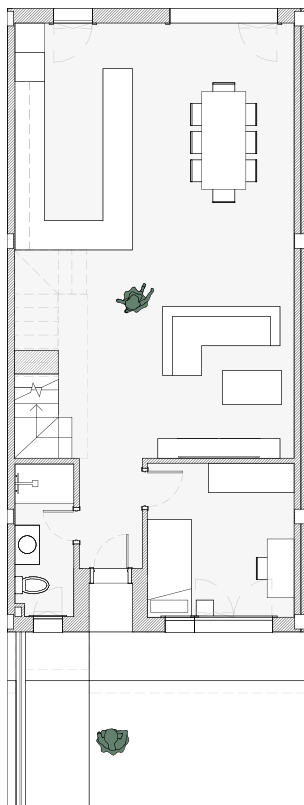
PLANTA BAJA
