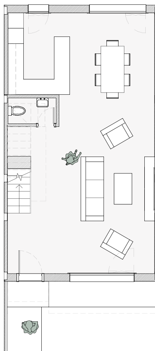
PLANTA BAJA
